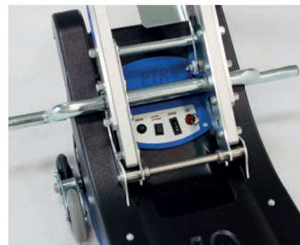
Bedienelement Basiseinheit
